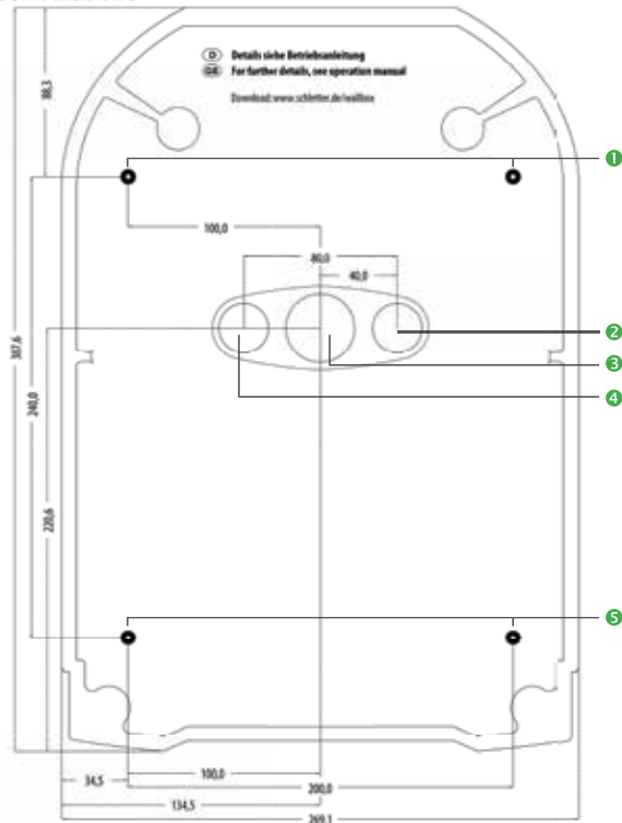
Bohrschablone
