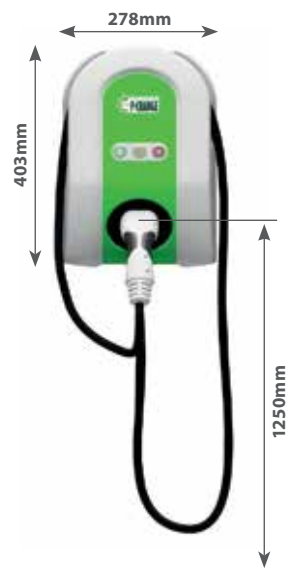
Abbildung 13: Montagehöhe
